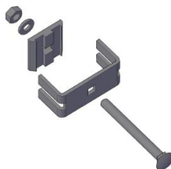
Комплект крепления №5/60 ПВД М8-120
