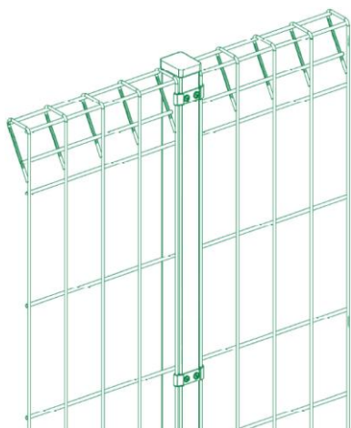
Крепление со скобой к столбу 50x40мм
