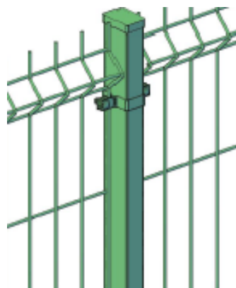
Комплект крепления №3 промежуточный 60x40 (60x60, 80x80)
